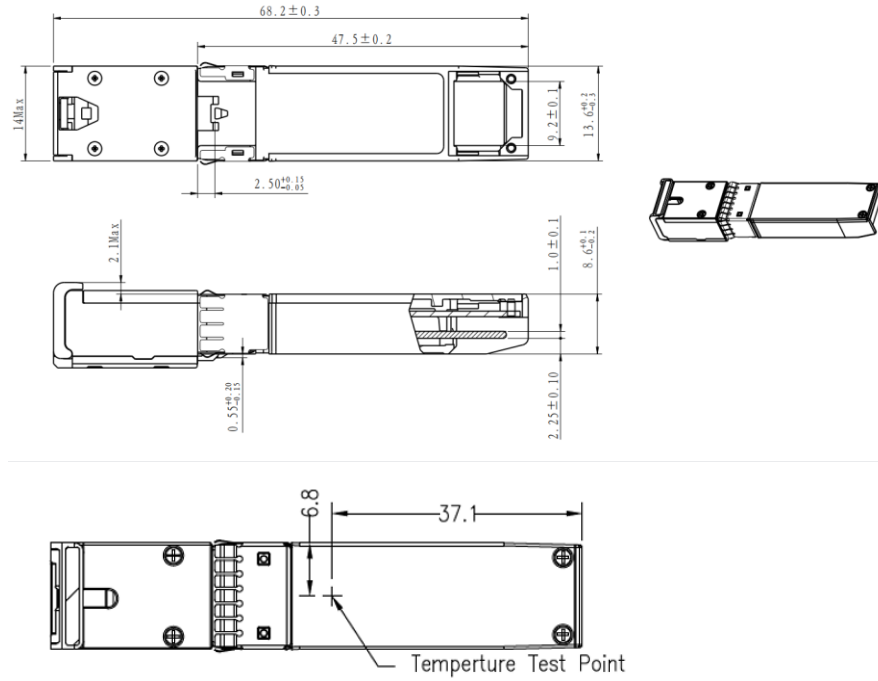
APCL52SCDSC1A
